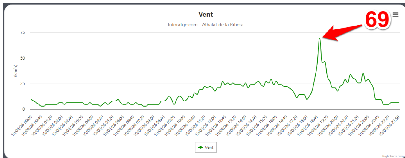
Ráfagas de viento máximas registradas en ALBALAT DE LA RIBERA el 10/08/26 (en km/h) https://inforatge.com/meteo-albalatdelaribera
